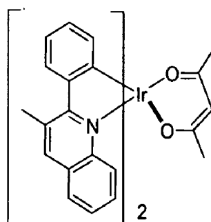
Ir(3-Mepq) 2 (acac)
