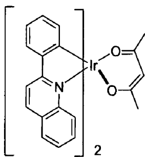
Ir(pq) 2 (acac)
