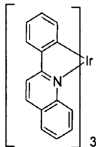
Ir(pq) 3
