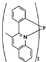
Ir(3-Mepq) 3
