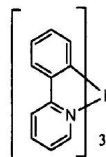
Ir(ppy) 3
