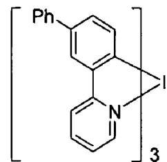
Ir(5-Phppy) 3
