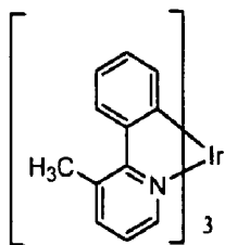
Ir(3-Meppy) 3
